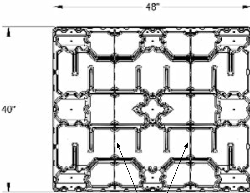
Ubicación de las barras de acero
